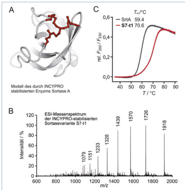
◀ Abb. 2: Beispiel der durch INCYPRO stabilisierten Sortase A. A, Modell der molekularen Struktur einer zyklisierten Sortase-A-Variante, basierend auf PDB-ID 1t2w. B, ESI-Massenspektrum der durch INCYPRO stabilisierten Sortase S7-t1 direkt nach der chemischen Quervernetzung. C, Schmelzkurven der Wildtyp-Sortase-A (SrtA, grau) und S7-t1 (rot) einschließlich der resultierenden Schmelzwerte.
